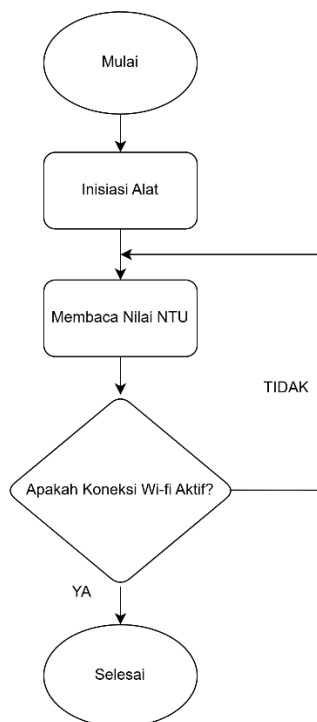
Gambar 4. Flowchart Pembacaan Turbidity Sensor
