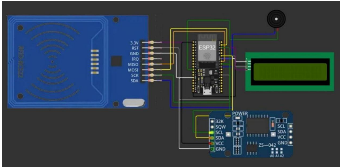
Gambar 6. Halaman Rangkaian Wokwi
