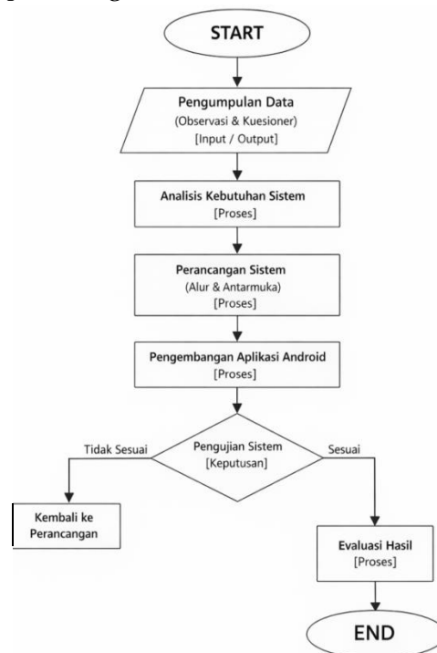
Gambar 1. Langkah-Langkah Penelitian
